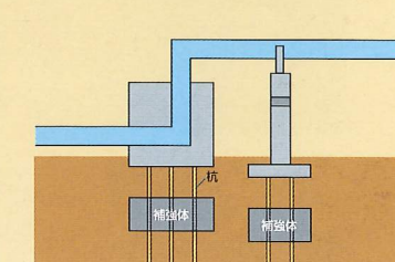
水管橋基礎
